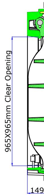
Section A-A
